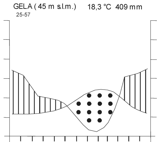
Fig. 2 – Diagramma termopluviometrico
